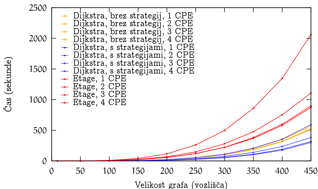
Slika 4.3: Trajanje računanja vseh najcenejših poti v grafu za Dijkstrin algoritem in pristop na osnovi ogrodja Etage .
