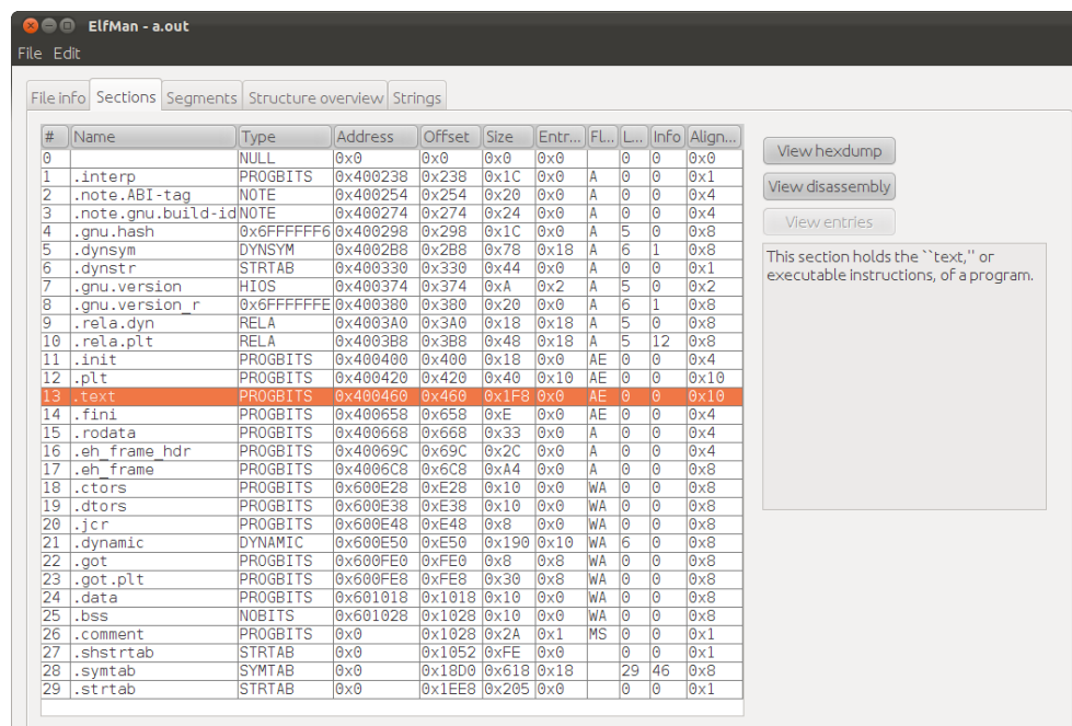
Slika 4.1: Zasloni posnetek pregleda sekcij.
