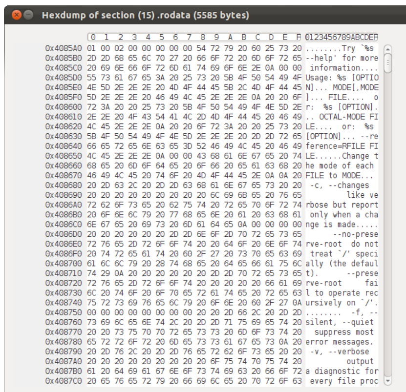
Slika 4.2: Zaslonski posnetek šestnajstiškega prikaza sekcije .rodata programa chmod . Na levi strani so prikazani pomnilniški naslovi posameznih vrstic, na desni pa znakovna predstavitev podatkov s kodiranjem ASCII.
