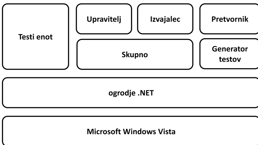
Slika 6: Struktura aplikacije
