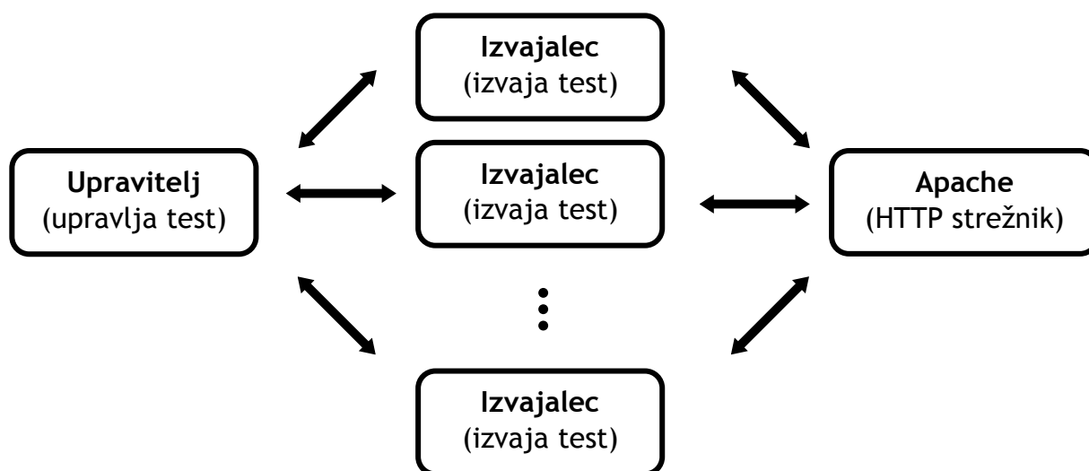
Slika 9: Postavitev aplikacije
