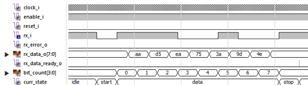
Slika 2.21: Primer ene periode notranje ure za potrebe RX in TX modula.
