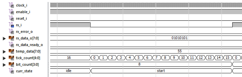
Slika 2.20: Primer branja enega bita v RX modulu.
