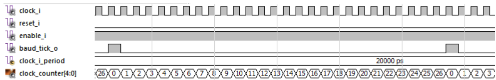
Slika 2.18: Primer ene periode notranje ure za potrebe RX in TX modula.
