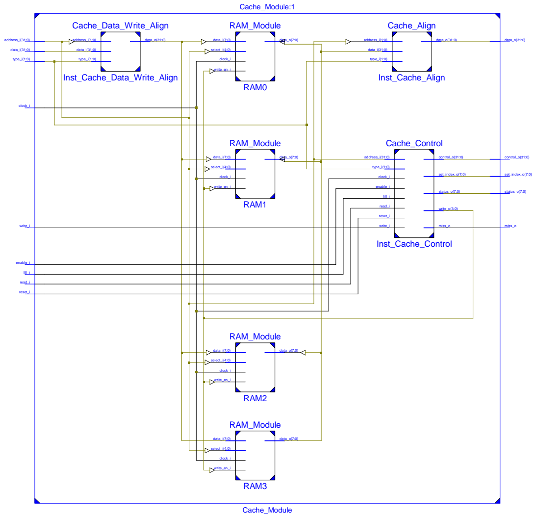
Slika 2.5: Shema RAM.
