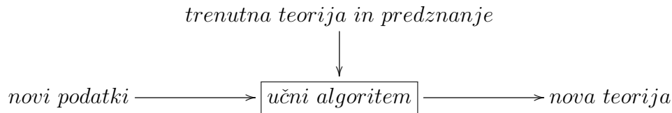
Slika 2.2: Inkrementalno učenje
