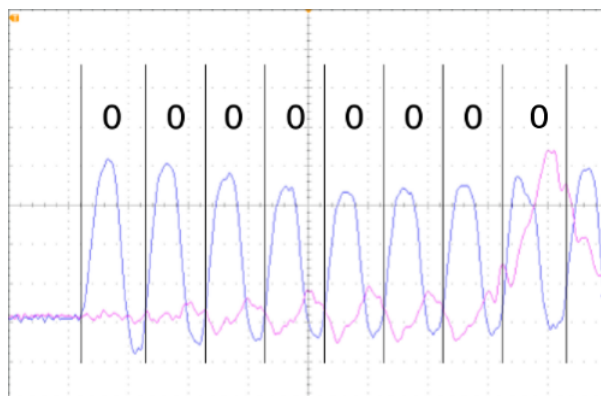
Slika 5.2: Posnetek signalov na QSPI linijah pri 100 MHz.
