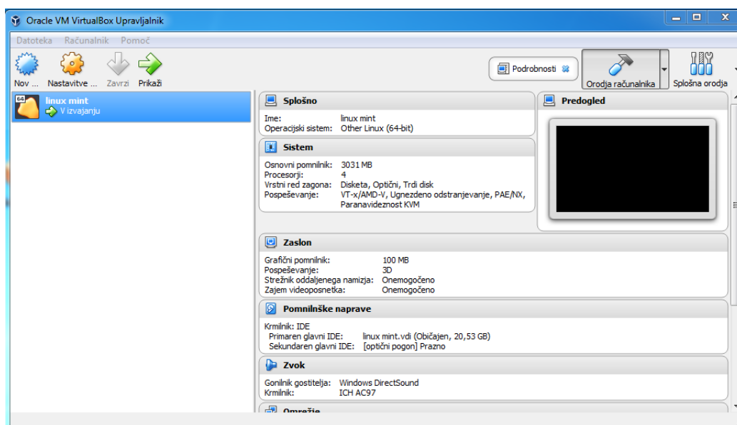
Slika 2.2: Program Virtualbox
