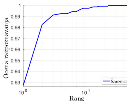
(b) Na semi-logaritmični skali prikazana CMC krivulja.
