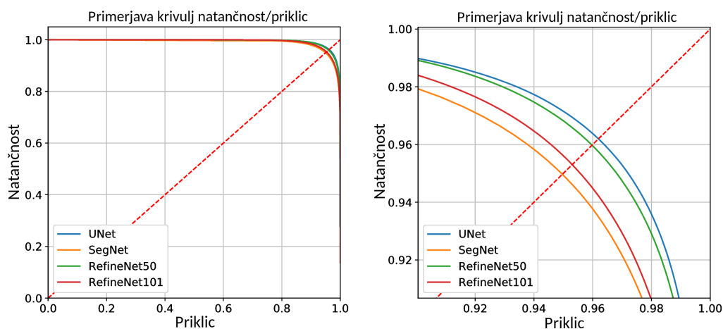
Slika 5.5: Prikaz krivulj natančnost-priklíc za testirane CNN modele. USS tukaj ni prikazana, ker metoda vrne le binarno masko segmentirane beločnice. Levi graf kaže celoten izris krivulje, ki ga dobimo s premikanjem segmentacijskega praga \Delta čez vse možne vrednosti, medtem ko desni graf prikazuje približno regijo levega grafa, kjer se vidijo majhne razlike med tehnikami. Rdeča pikčasta črta prikazuje operativne točke, kjer sta natančnost in priklíc enaka.
