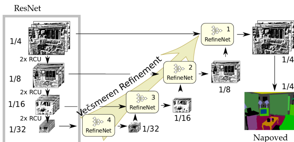
Slika 3.17: Prikaz arhitekture RefineNet [95]. Kodirnik je sestavljen iz mreže ResNet, pri čemer je vsak nivo map značilnik eden izmed vhodov v istoležni RefineNet blok (drugi vhod v RefineNet blok je izhod RefineNet bloka nižjega nivoja).
