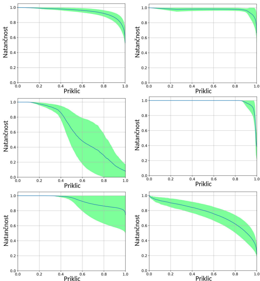
Slika 6.4: Povprečne krivulje natančnost-priklic (s standardnim odstopanjem), ki jih generiramo med ovrednotenjem SegNet modela z uporabo THS strategije in 4-kratnega prečnega preverjanja. Grafi prikazujejo rezultate (od leve proti desni, od zgoraj navzdol): periokularne regije, beločnice, kantusa, šarenice, zenice ter trepalnic.
