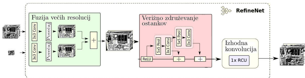
Slika 3.19: Natančnejši prikaz RefineNet bloka [95]. Na vhod dobimo mape značilnk iz istoležnega nivoja in iz RefineNet bloka nižjega nivoja. Oba vhoda povečamo na isto velikost in ju seštejemo. Verižno združevanje ostankov zajame kontekst ozadja.
