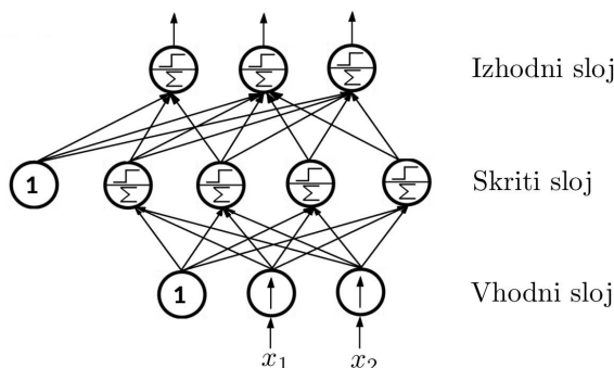
Slika 3.5: Večslojni perceptron [81].
