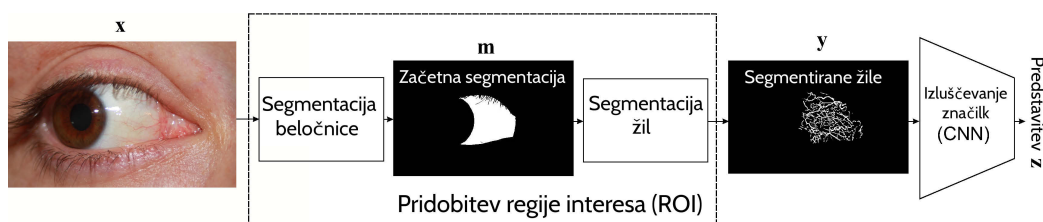
Slika 5.1: Prikaz predlaganega bločnega diagrama, ki opisuje algoritem za razpoznavanje na podlagi beločnice. Najprej so z uporabo dvo-fazne segmentacijske procedure segmentirane vaskularne strukture v predelu beločnice. Verjetnostna mapa vaskularnih struktur je nato podana CNN modelu (imenovanemu ScleraNET), ki izlušči diskriminativne značilke. Slednje so uporabljene za izračun ujemanja.
