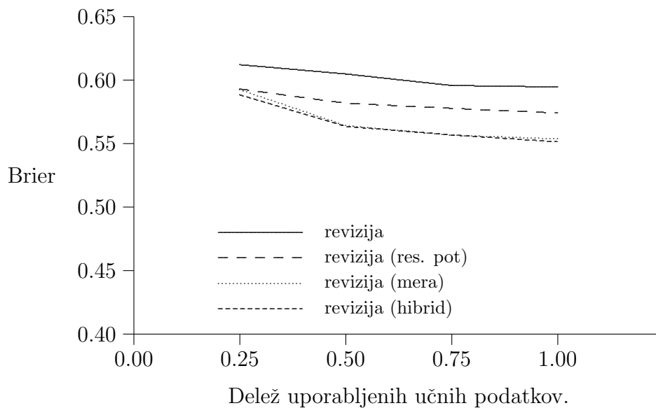
Slika 5.3: Učne krivulje metod revizije na modelu Mp pri razdelitvi podatkov na 50% učnih in 50% testnih in m=5 .
