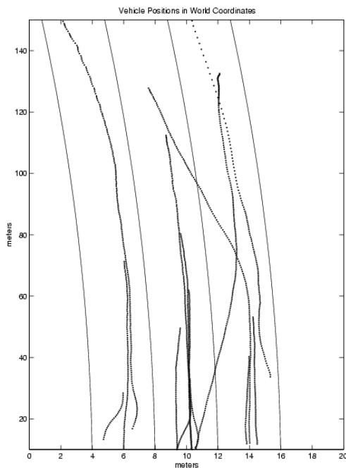
Slika 7: Projekcija sledi iz slike 6 na tloris ceste
