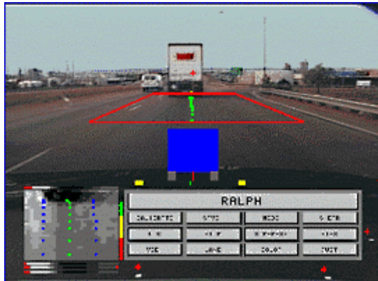
Slika 8: Sistem za ugotavljanje prečne (lateralne) lege vozila spremlja trapezno območje cestišča pred vozilom
