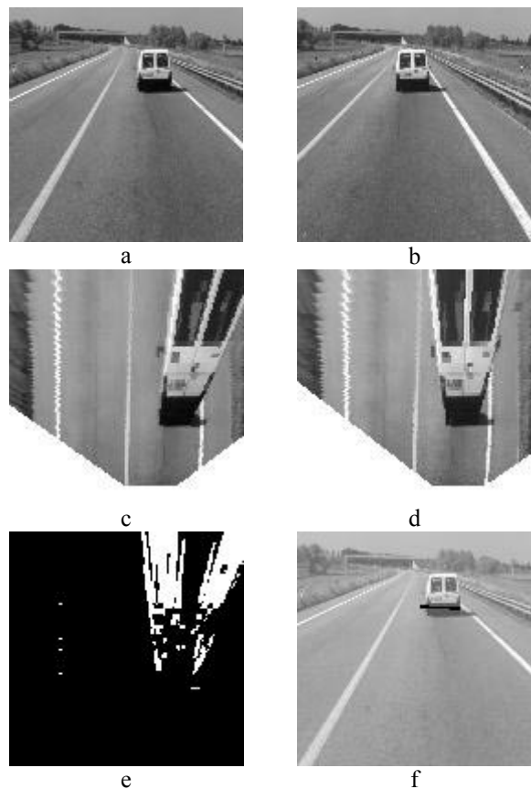
Slika 10: Delovanje sistema GOLD: (a) slika iz leve in (b) desne kamere, odpravljena perspektivna projekcija (c) leve in (d) desne slike, (e) razlika med slikama c in d, (f) označeno mesto na sliki, kjer je ovira (vozilo)
